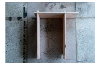
② 片方の側板に棚板を差し込む 天板の木表を上面に、片方の側板を立てかけた状態で天板2枚を差し込む。
