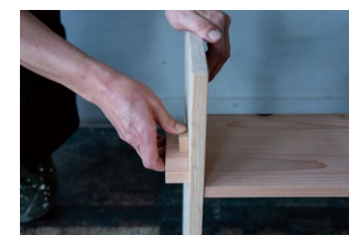
⑤ 仕上げ 本体を起こしてクサビが動かなくなるところまで差し込み完成。*金槌などを使用する場合はクサビより大きめの板や本などを噛ませてください。本体の凹みの原因になります。
