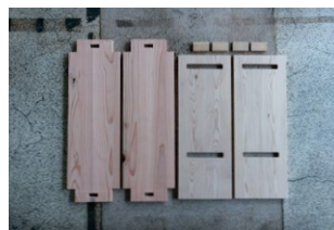
① 8つのパーツ 棚板2枚・側板2枚・クサビ4つ
